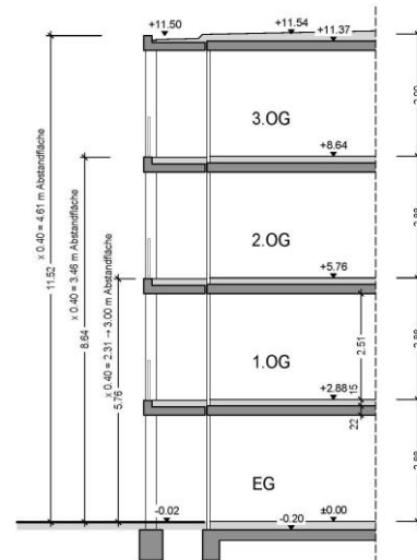
SYSTEM - SCHNITT
