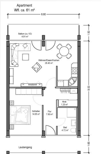
SYSTEM - GRUNDRISS 2-Achsen alt. Senioren-Whg. mit barrierefreies Bad
