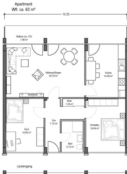
SYSTEM - GRUNDRISS 3-Achsen Familie 3-Z-K-B oder 4-Z-K-B
